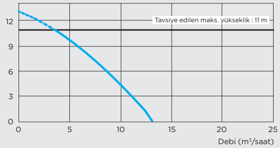
Debi performansı
